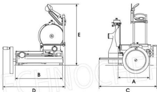
F 350 VOLANO
