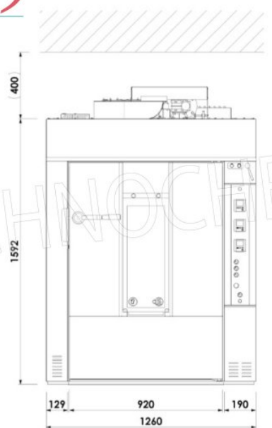
VISTA FRONTALE
